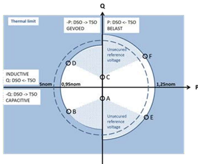
Figuur 53: Toegelaten werkingszone voor de spanningsregelaars van de HS/HS-transformatoren
