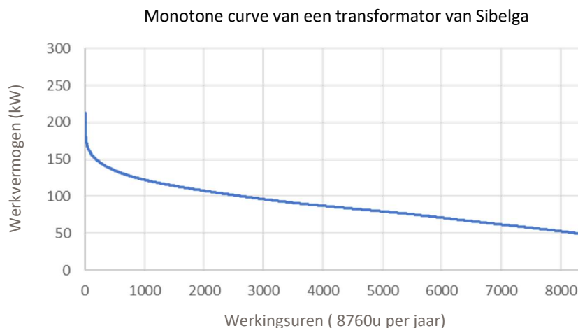
Figuur 3: Monotone curve van een transformator van Sibelga
