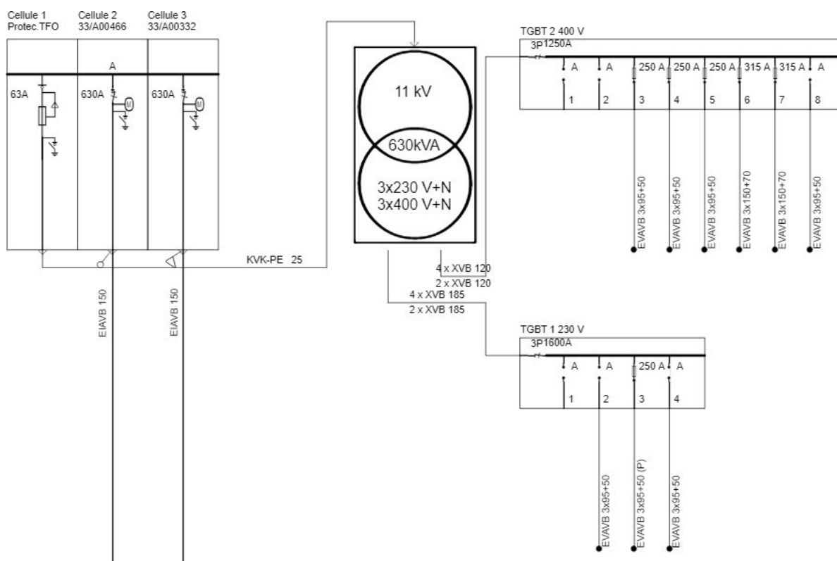
Figuur 23: Uittreksel uit de GIS-database van Sibelga – Eendraadsschema van een netcabine
