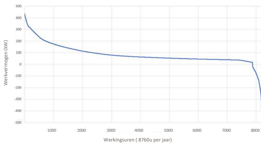
Figuur 4 - Monotone curve van een transformator van Sibelga met afvoer
