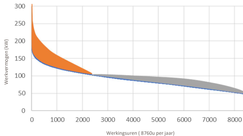
Figuur 5: Impact van nieuwe toepassingen op de monotone curve van een transformator van Sibelga
