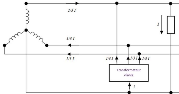
Figuur 41 - Principeschema van een zigzagtransformator
