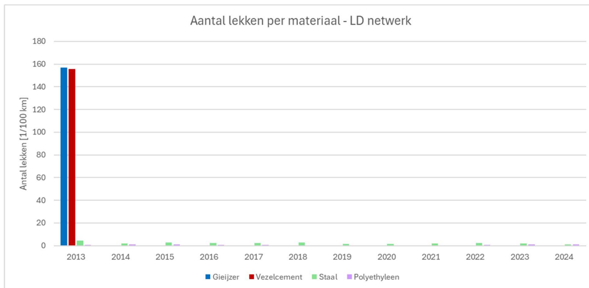
Figuur 3: evolutie van het aantal lekken per materiaal - LD-net
